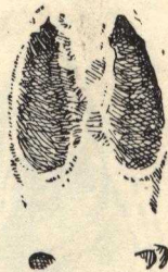
След лося. Задняя нога полностью покрывает след передней.
