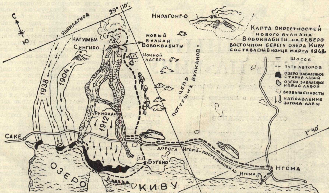
На этой карте вы видите направление потоков лавы при извержении нового вулкана Вовокwabити, а также при извержениях других вулканов в 1904, 1912 и 1938 годах.
